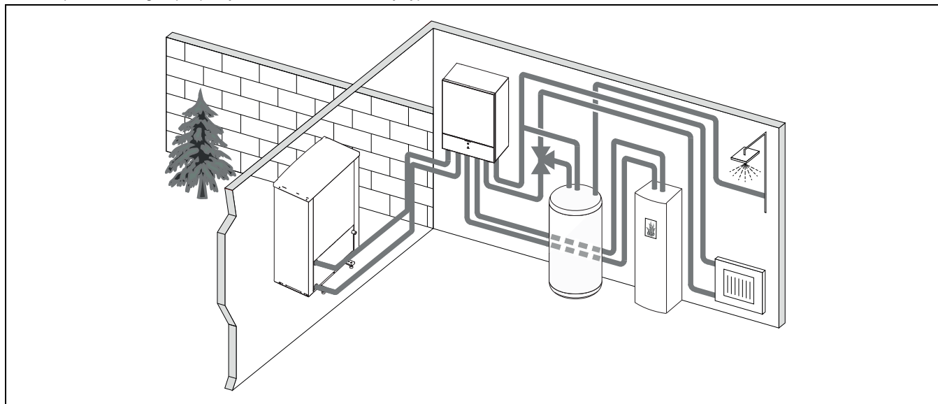
Obr. 3 Tepelné čerpadlo AirX 400, vnitřní jednotka Airbox S bez elektrické pomocné topné tyče, externí zásobník teplé vody a externí dohřev
