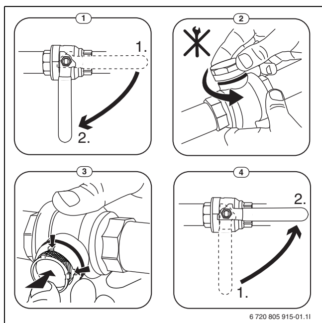
Obr. 8 Čištění sítka
