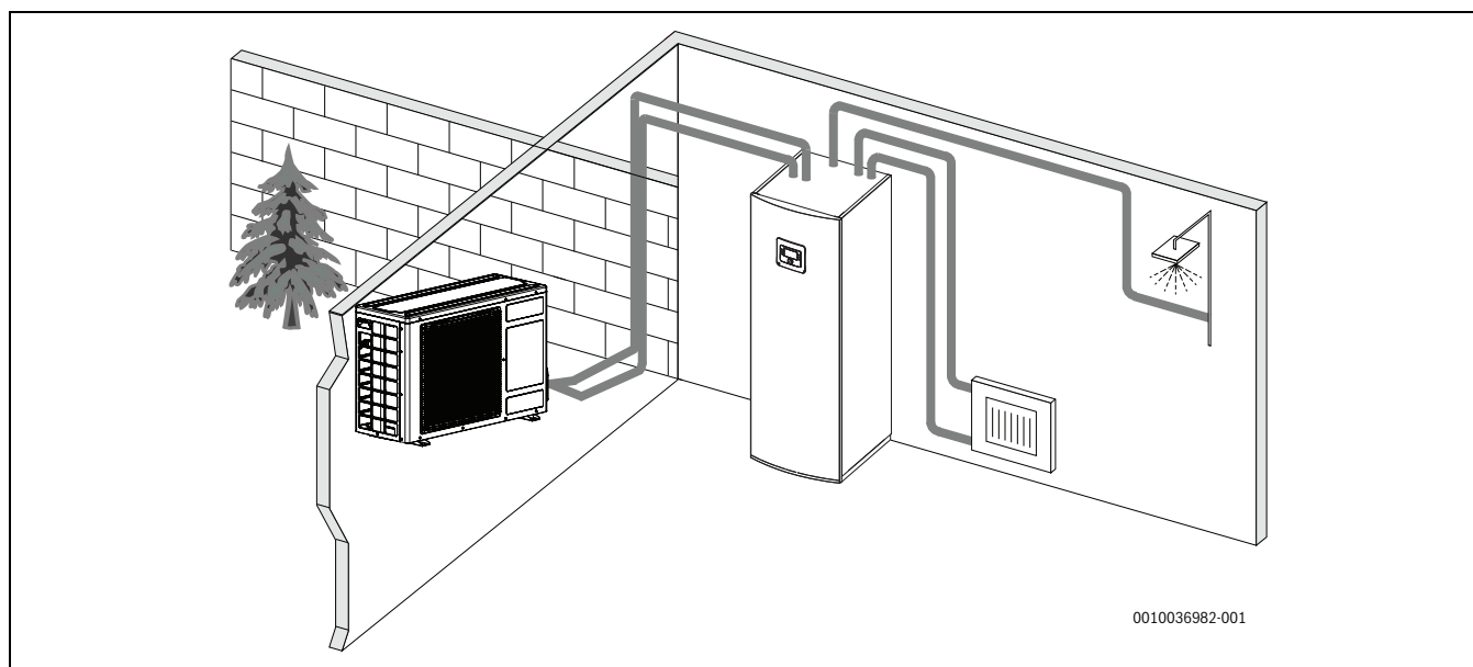
Obr. 2 Tepelné čerpadlo pro venkovní jednotku, vnitřní jednotku AWS M s integrovaným zařízením na přípravu teplé vody a elektrickou pomocnou topnou tyčí
